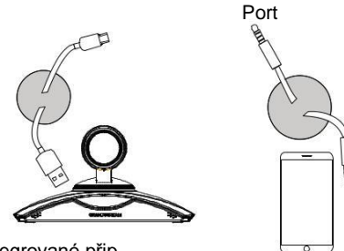
Připojení mobilního zařízení: GAC2500 (stan- dardní připojení) se připojuje k mobi- lnímu zařízení pomocí kabelu 3,5 mm samec-samec.
