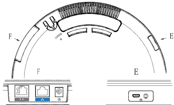
Kaskáda LAN port Napájecí port
